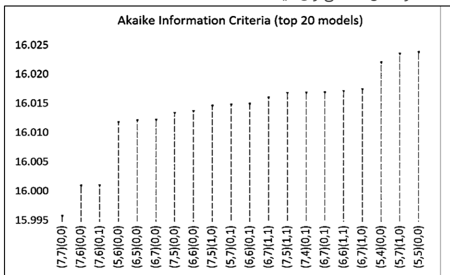
شکل ۳- بیست مدل برتر روش تفاضل‌گیری با کوچکترین معیار اطلاعاتی آکائیک (AIC) برای شاخص صنایع غذایی
