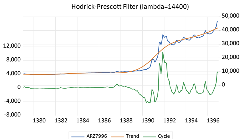
نمودار ۱. فیلتر هدریک - پرسکات
