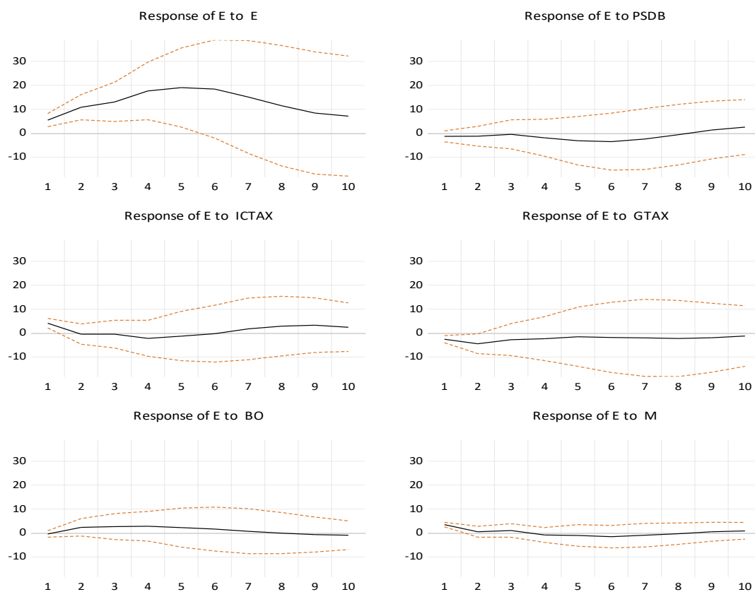
نمودار ۳. توابع واکنش آنی جریان نابرابری درآمدی
