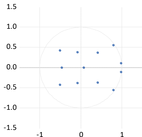
مدل نامانی اقتصادی Inverse Roots of AR Characteristic Polynomial
