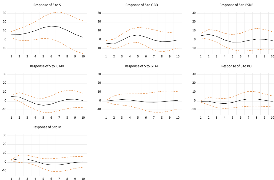
نمودار ۴. توابع واکنش آنی نامانی اقتصادی
