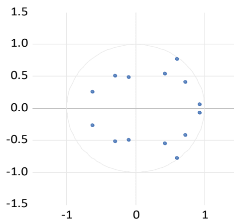
مدل نابرابری درآمدی Inverse Roots of AR Characteristic Polynomial
