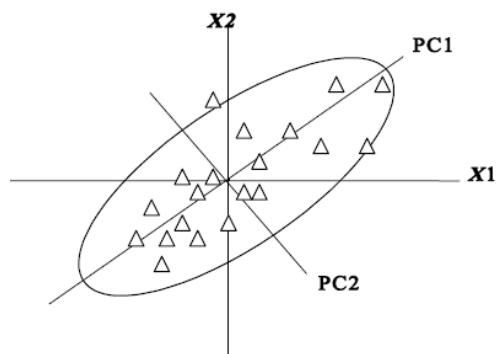
نمودار ۱. تبدیل داده‌ها به مؤلفه‌های اصلی
